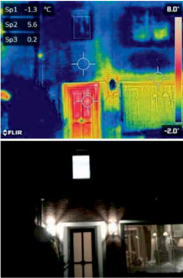
Warmtescan van een goed geïsoleerd huis, de voordeur lekt de meeste warmte
